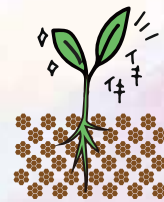
団粒構造
