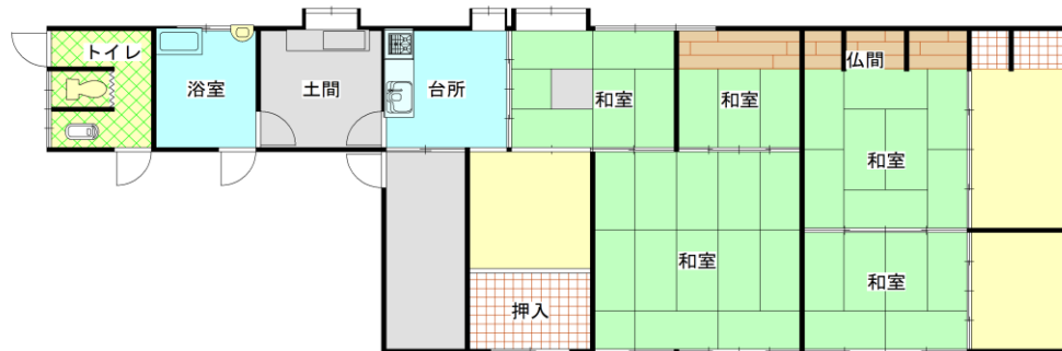
1階平面図
