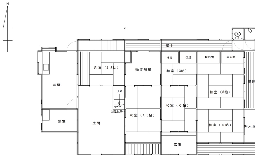
平屋 間取り図 (木造)
