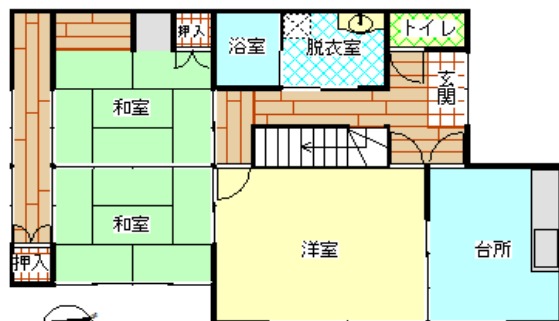
1階 平面図
