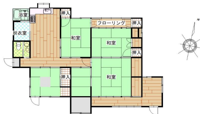
1 階平面図
