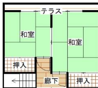
2階平面図
