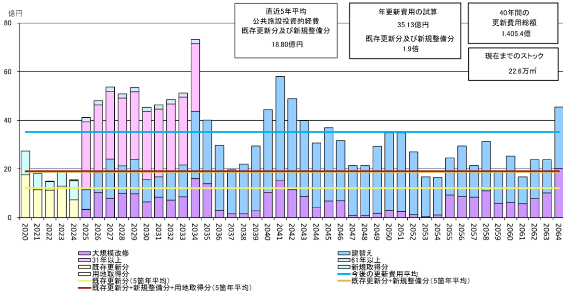
図表 公共構築物の更新費用試算結果
