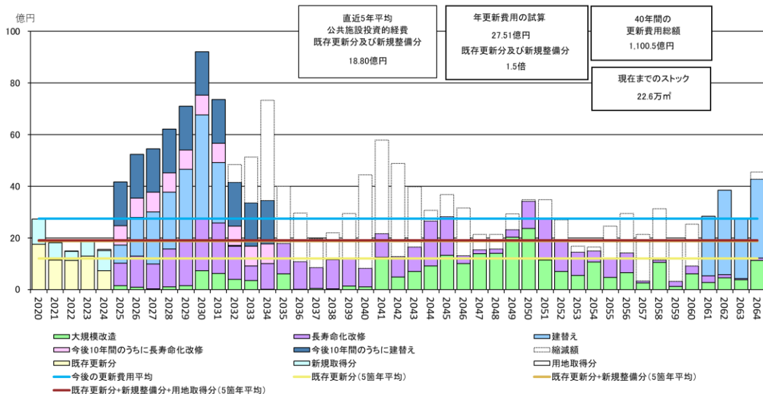
図表 公共構築物の更新費用試算結果（長寿命化等考慮）
