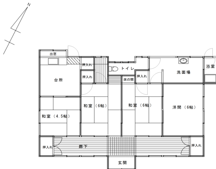
間取り図 平屋（和室）
