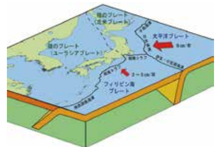
▲日本付近のプレートの模式図
