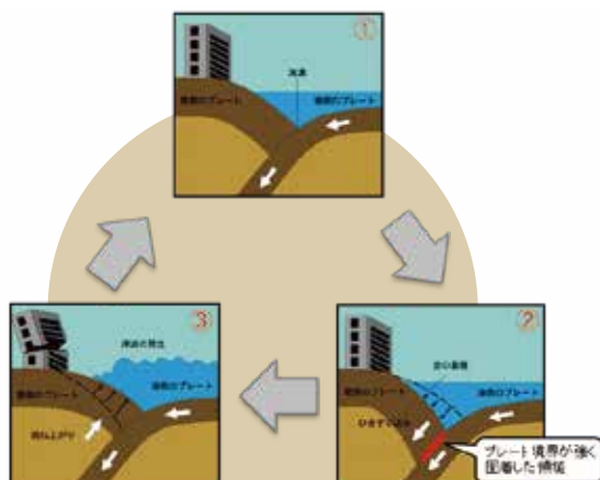
▲南海トラフ地震発生メカニズムの概念図
